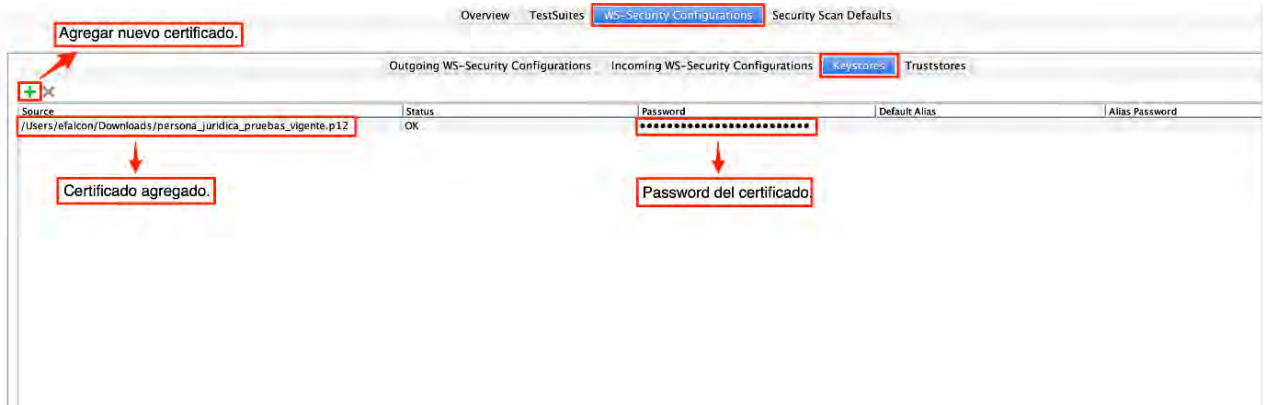
Ilustración 3. Configuración keystore
